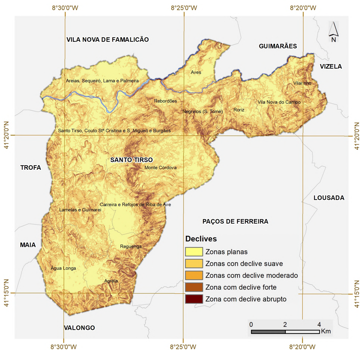
Figura I.5 - Carta de declives.
