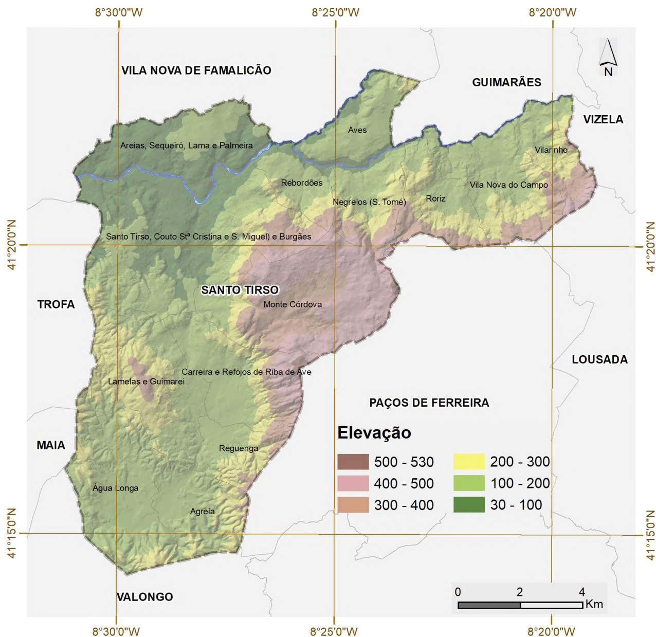
Figura I.3 - Modelo digital do terreno.
